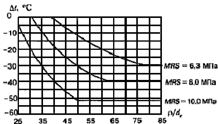
Рисунок 4 - Максимально допустимый отрицательный температурный перепад в зависимости от отношения радиуса упругого изгиба к наружному диаметру газопровода
