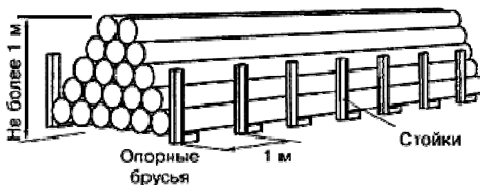
Рисунок 9 - Хранение отдельных труб в штабеле Высота штабеля при предполагаемом сроке хранения свыше двух месяцев не
