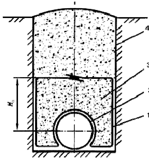
Рисунок Г.1 - Схема балластировки газопровода
