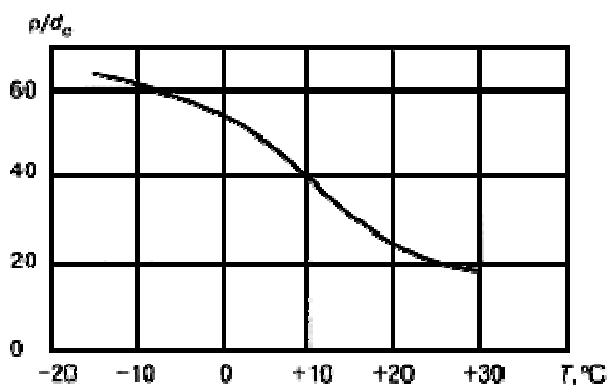
Рисунок 18 - Зависимость отношения радиуса упругого изгиба газопроводов R к наружному диаметру трубы d_g от температуры окружающего воздуха T при монтаже и укладке газопроводов
