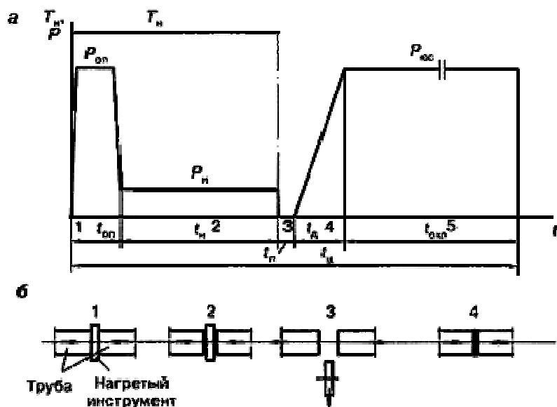
а - диаграмма изменения во времени t давления на торцах P и температуры нагретого инструмента T_H ; б - последовательность протекания процесса сварки; 1 - оплавление торцов; 2 - нагрев концов труб; 3 - вывод нагретого инструмента (технологическая пауза); 4, 5 - осадка и охлаждение стыка
